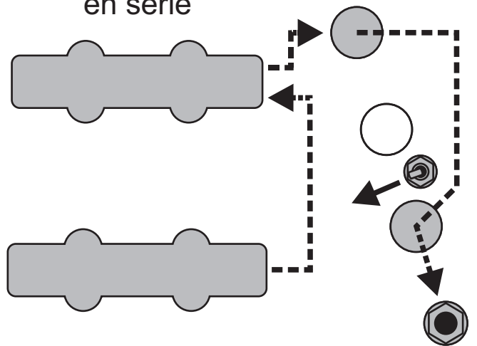
Pastillas en serie
